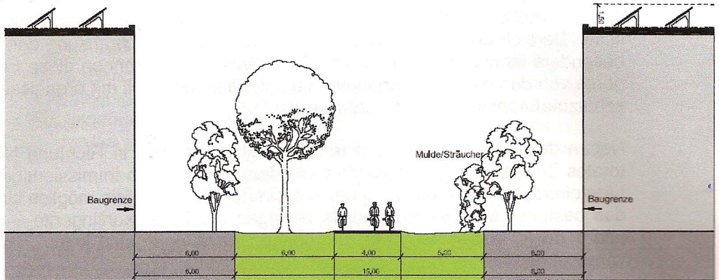
Schnitt: Schlattweg (Ost-West-Verbindung) mit öff./priv. Grünsaum
